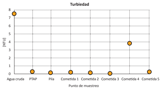
Figura 3. Se observa el efecto en el aumento de la concentración media de dos días de muestreo de Al, Fe y Mn y el aumento en turbiedad (NTU) en la cometida 4 debido al evento de coloración registrado en el muestreo y concentraciones constantes en los muestreos en las cometidas bajo condiciones de operación normal
